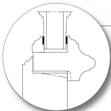
Moulure grand cadre
