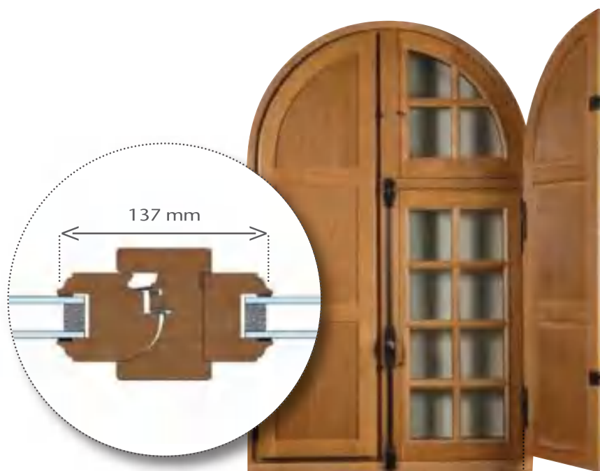
Ferrage par paumelles
